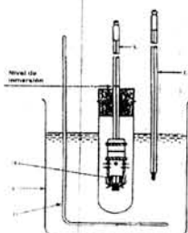
Figura- Aparato I para determinación de punto de fusión
